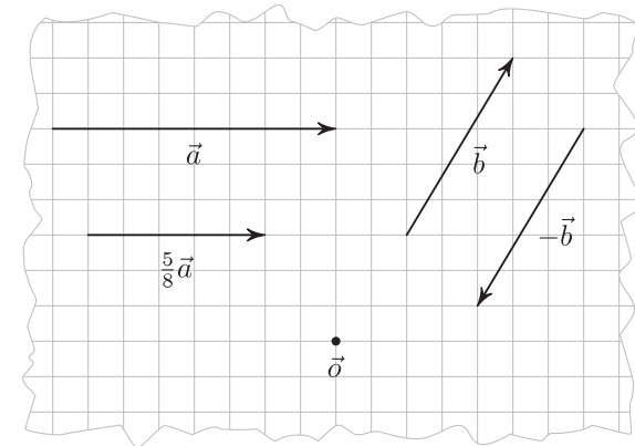
Abb 5.1 Illustration der Skalarmultiplikation und Inversion.
