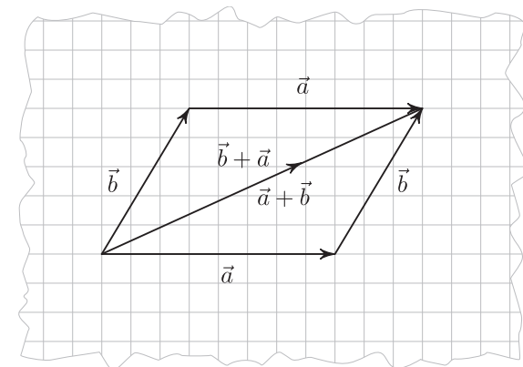
Abb 5.2 Addition zweier Vektoren und Illustration des Kommutativgesetzes. 7. März 2012
