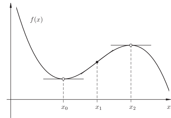
Abb 11.3 Bei x_0 ein lokales Minimum, bei x_1 ein Wendepunkt, und bei x_2 ein lokales Maximum.
