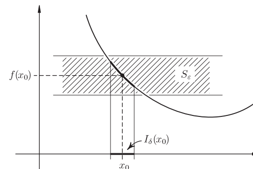
Abb 11.1 Geometrisch Deutung der Stetigkeit für den Fall D \subset \mathbb{R} und f reell: Zu jedem beliebig schmal vorgegebenen Streifen S_\varepsilon = \{(x, y) | f(x_0) - \varepsilon < y < f(x_0) + \varepsilon\} gibt es ein Intervall I_\delta(x_0) := \{x | x_0 - \delta \leq x \leq x_0 + \delta\} , so dass der Graph über diesem Intervall innerhalb dieses Streifens verläuft.
