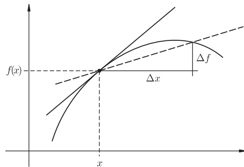
Abb 11.2 Geometrische Deutung der Ableitung. Es ist f'(x) = \lim_{\Delta x \rightarrow 0} \frac{\Delta f}{\Delta x} .
